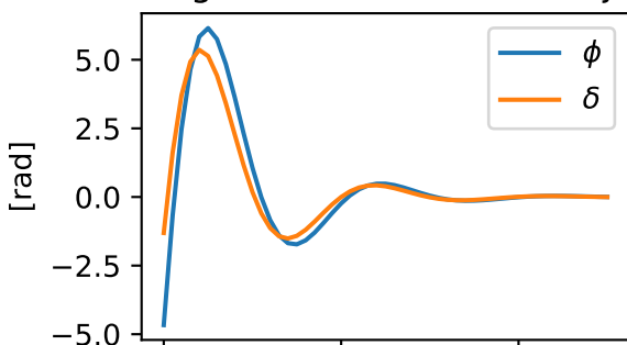
Eigenvalue: -0.402+0.000j
