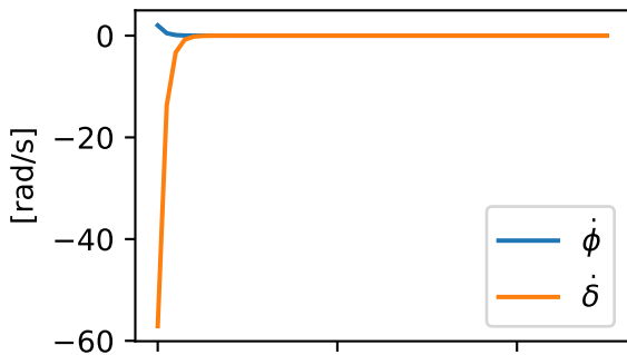
Eigenvalue: -1.292+3.209j
