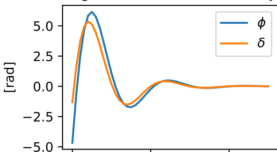
Eigenvalue: -1.292-3.209j
