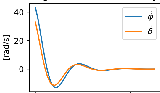
Eigenvalue: -0.402+0.000j
