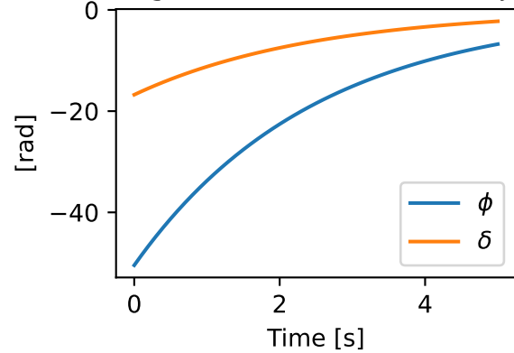
Eigenvalue: -0.402+0.000j
