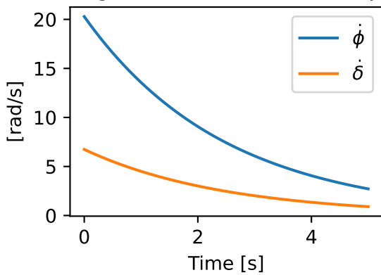
Eigenvalue: -0.402+0.000j
