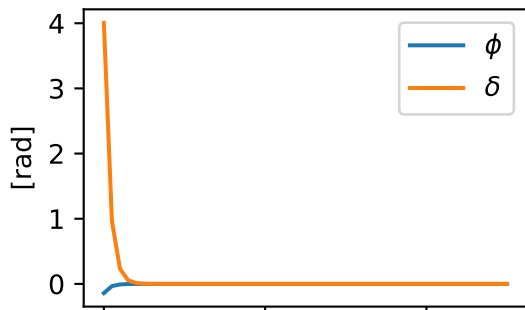
Eigenvalue: -1.292+3.209j
